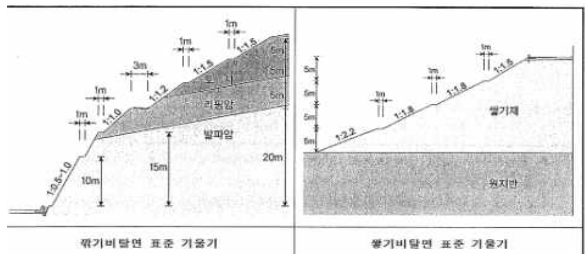
쌓기비탈면 표준 기울기
