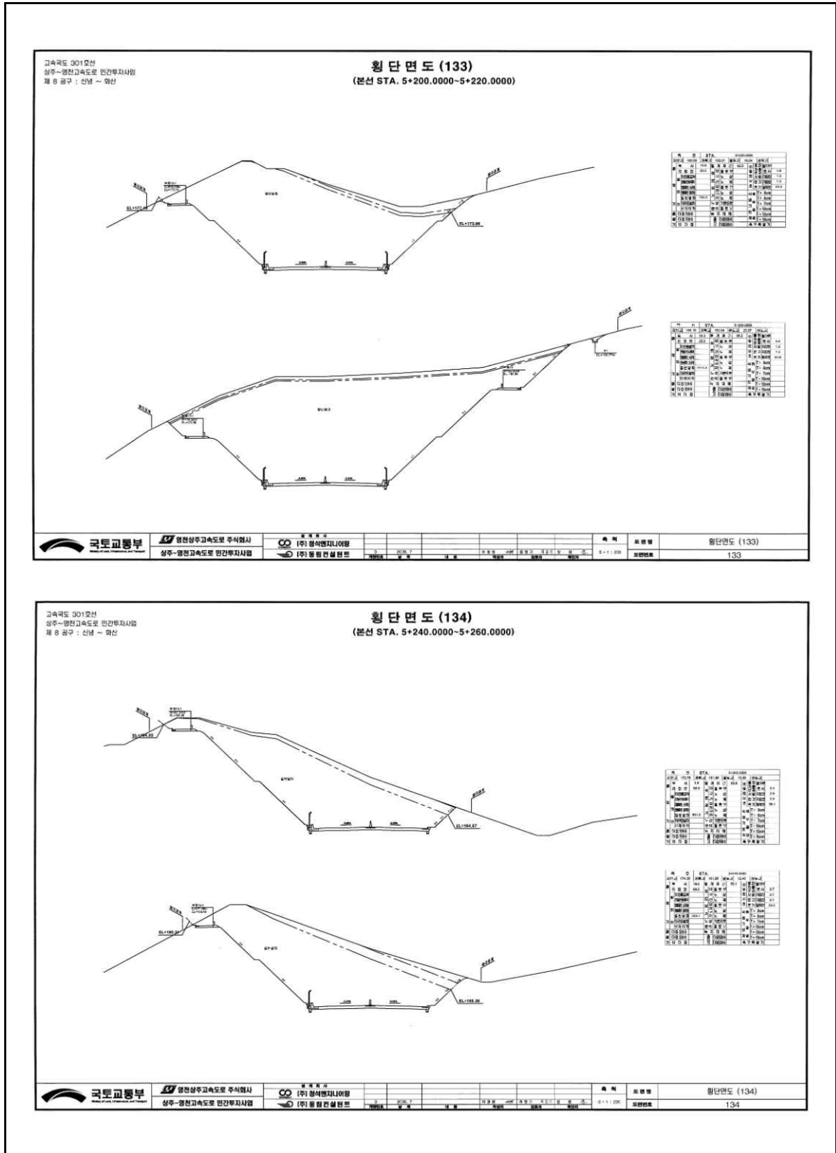
【그림 47.1.5】 표준형단면도
